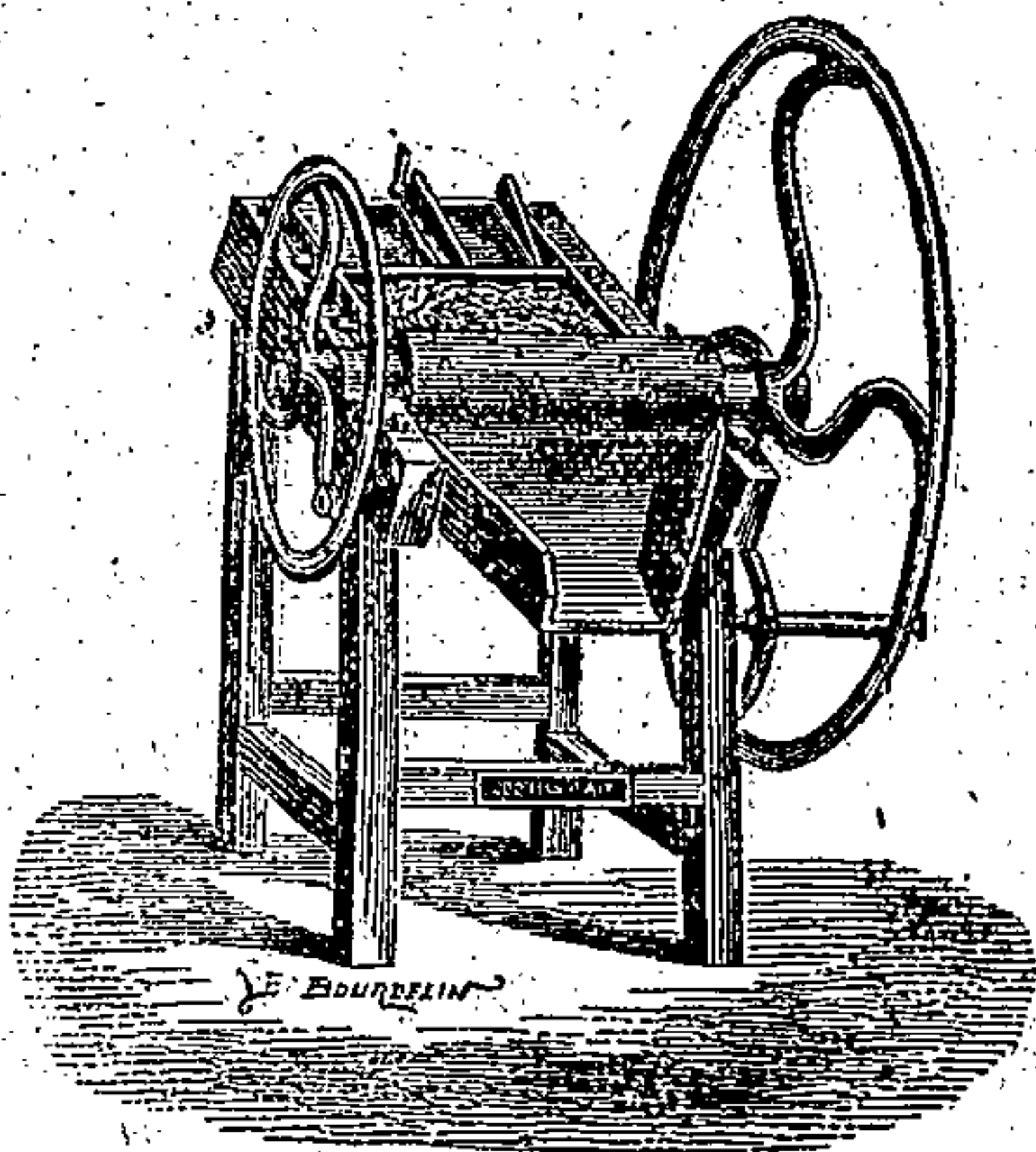
Moulin à Tourteaux.
