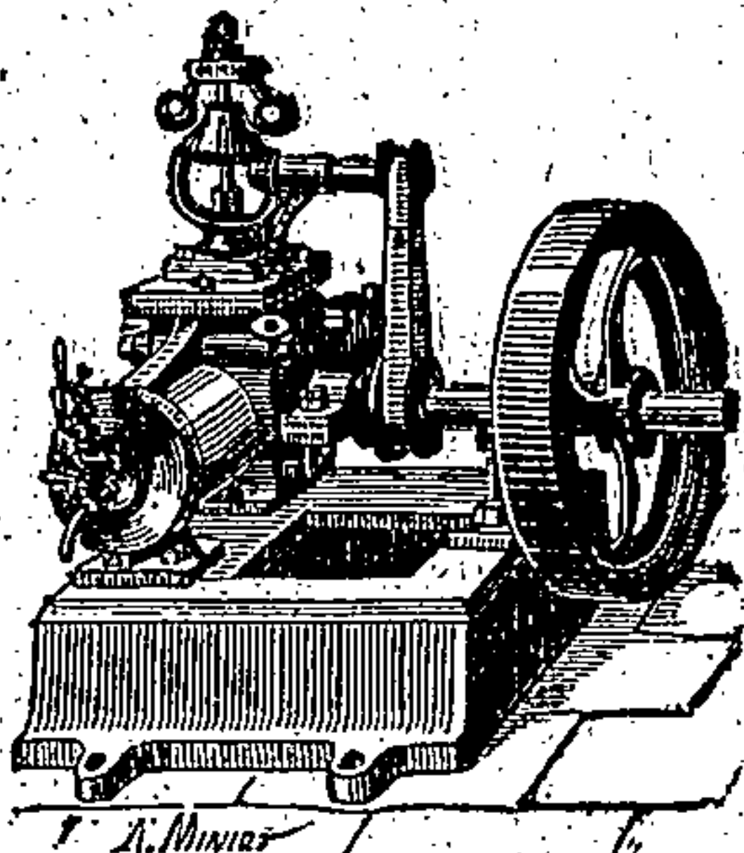
Machine à vapeur à détente variable Moteur rationnel.
