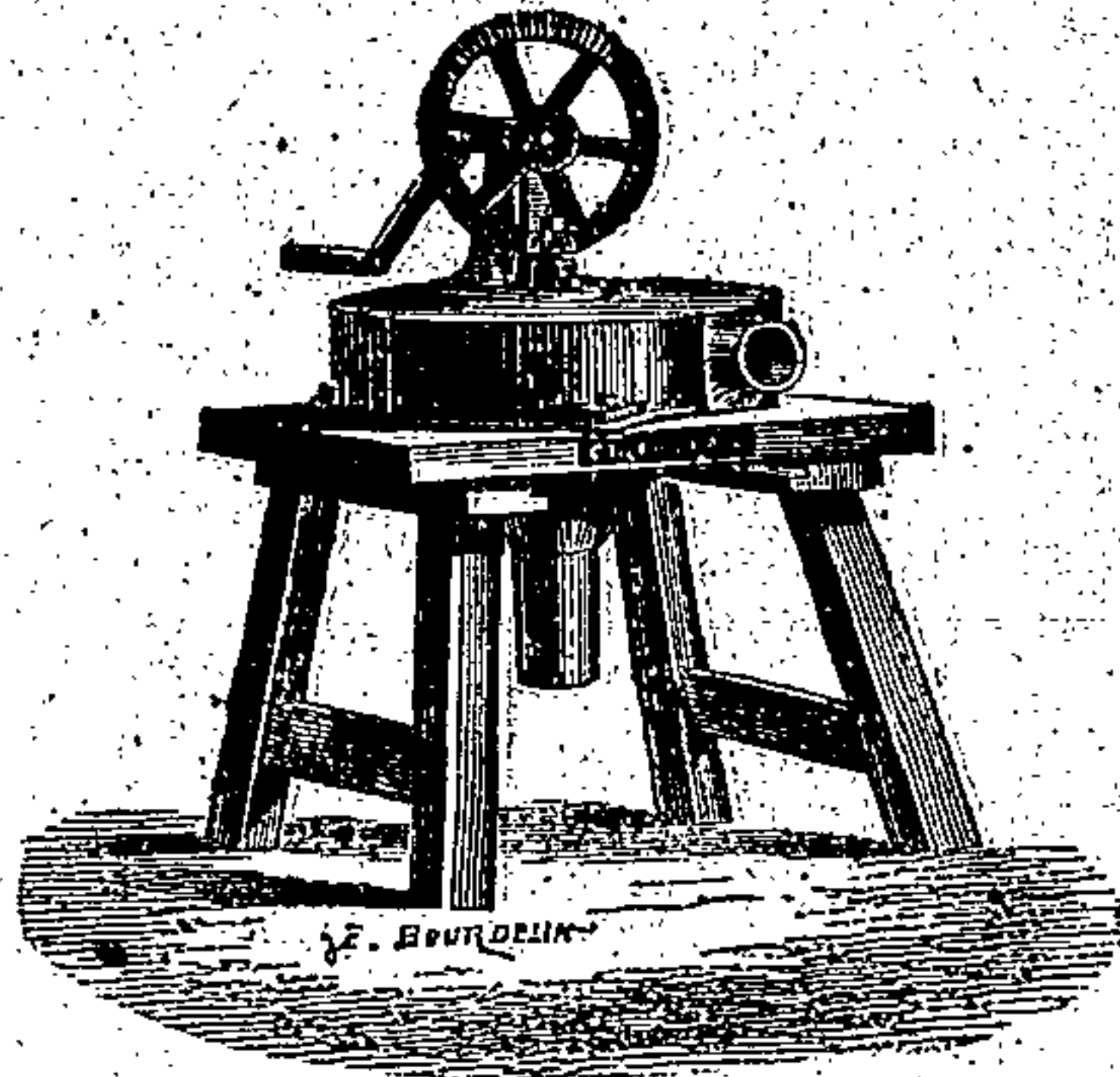
Aspirateur pour l'acide carbonique des cuves vinaires
