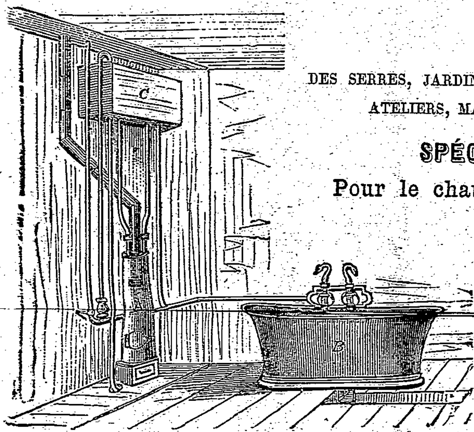
INSTALLATION D'UN APPAREIL THERMOSIPHON POUR CHAUFFAGE DE BAINS
