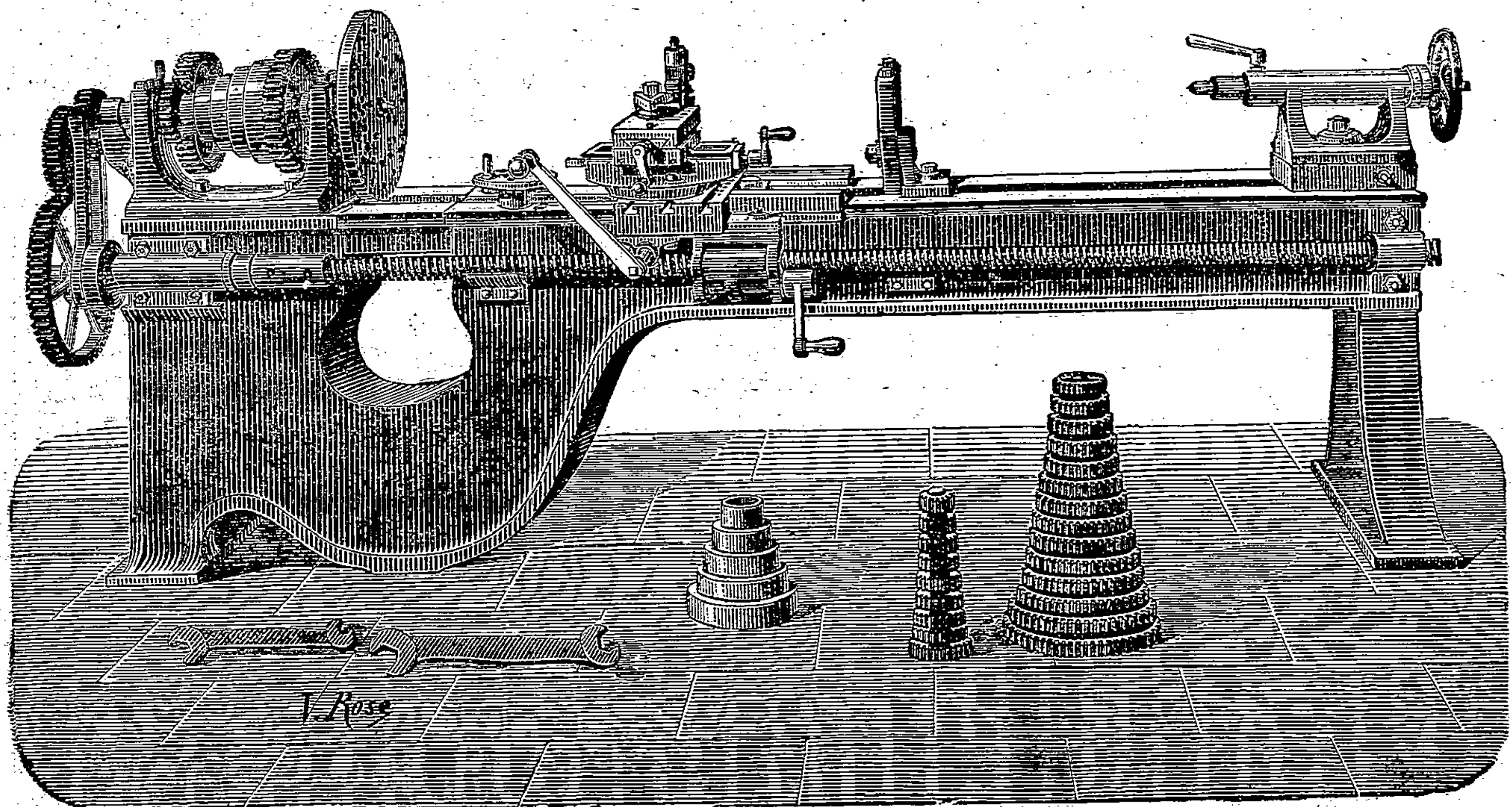
TOUR PARALLÈLE POUR FILETER & CYLINDRER MÉCANIQUEMENT PAR VIS — PEUT ALÉSER DE GRANDS DIAMÈTRES
