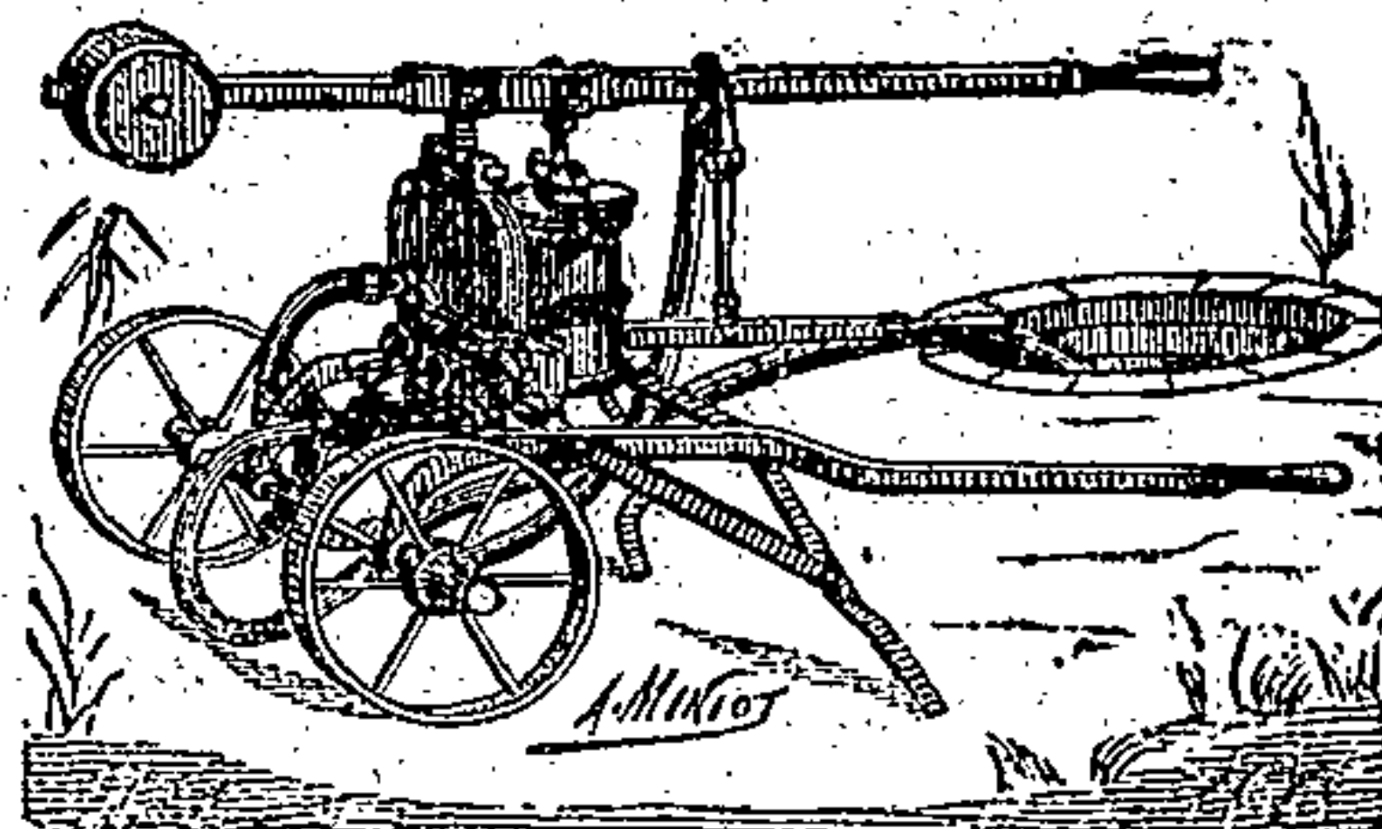
Nouvelle pompe pour tous usages : Arrosage, purin, épuiement, transvasement des vins, etc. Débit 6.000 litres par heure.
